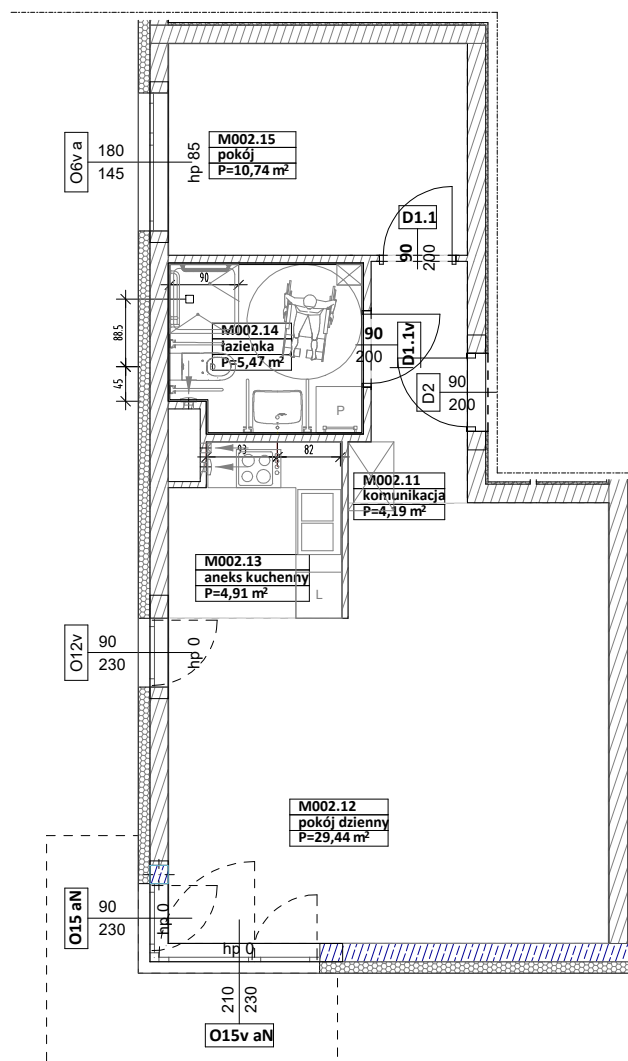
BUDYNEK 6MW-3
